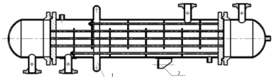
图 A.1 浮头式换热器
