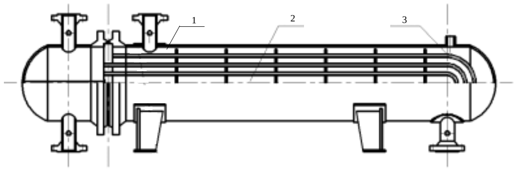
1—内导流筒；2—中间挡板；3—U 型换热管
