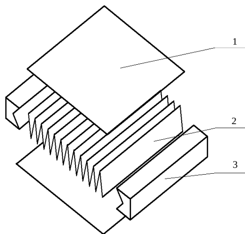
1—平板；2—翅片板；3—侧条
