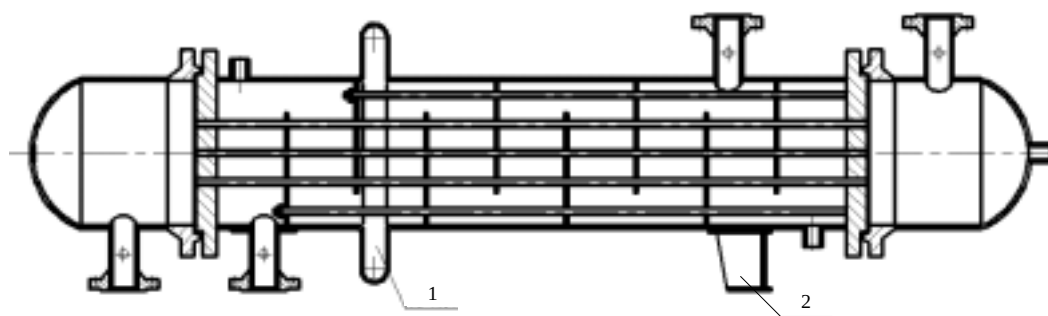
图 A.2 立式固定管板式换热器
