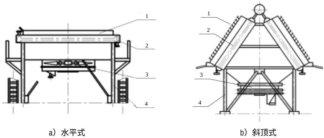
1—百叶窗；2—管束；3—风机；4—构架
