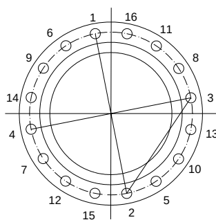
图 D.1 换热设备热紧、冷紧顺序
