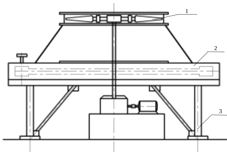
1—风机；2—管束；3—构架
