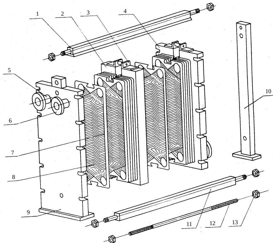
1—上导杆；2—中间隔板；3—滚动机构；4—活动压紧板；5—接管；6—法兰；7—垫片；8—板片 9—固定压紧板；10—支柱；11—下导杆；12—夹紧螺柱；13—螺母
