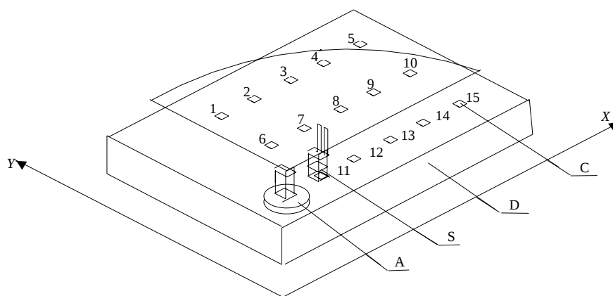
A - 发射器；S - 探测器；C - 测量点；D - 测量平板
