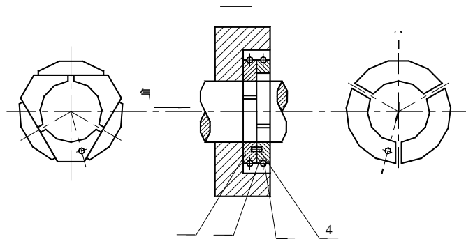
1 - 三瓣式；2 - 六瓣式；3 - 弹簧；4 - 圆柱销
