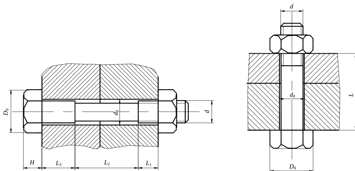
图L.1 螺栓连接
