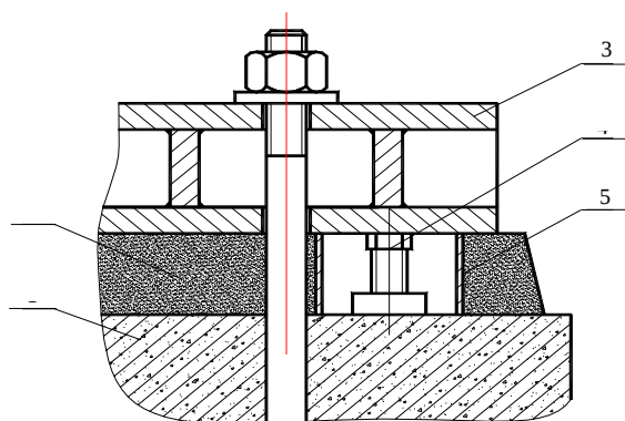
1 - 基础；2 - 二次灌浆层；3 - 设备底座；4 - 千斤顶(垫铁)；5 - 模板
