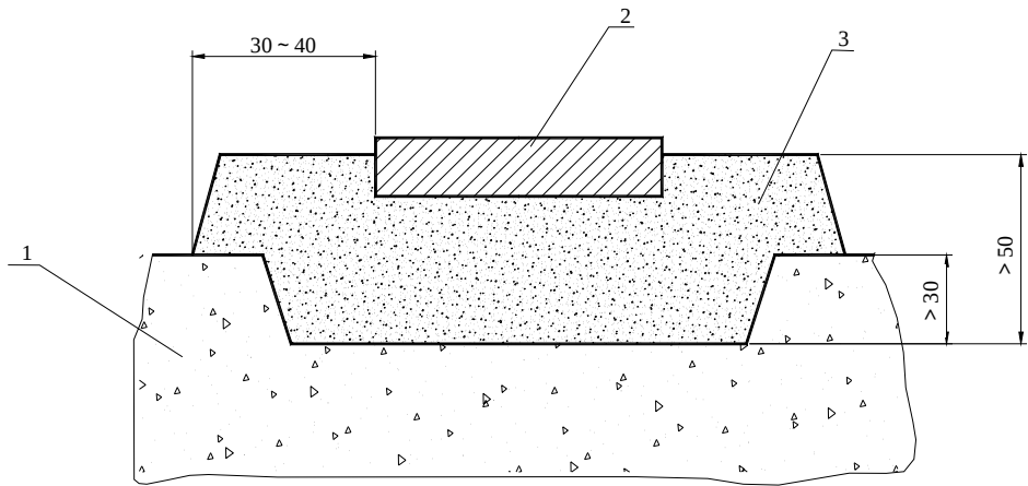
1 - 基础；2 - 垫铁；3 - 水泥砂浆
