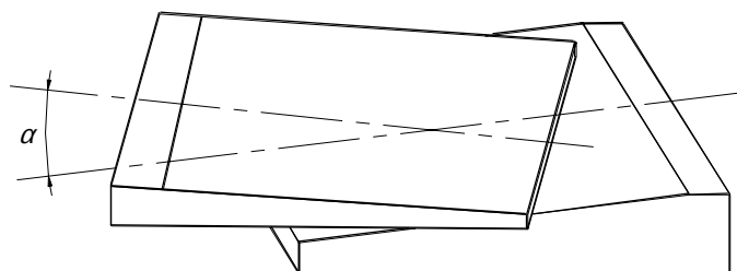
图2 斜垫铁放置位置示意
