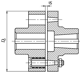
图18 弹性套柱销联轴器
