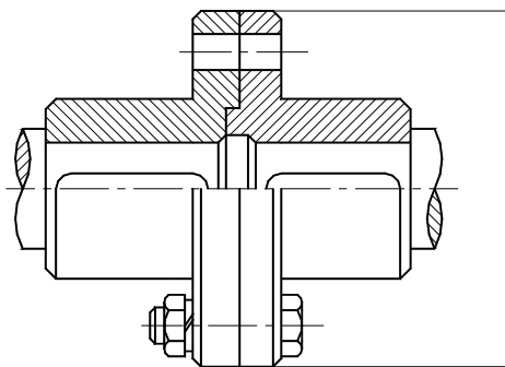
图15 凸缘联轴器
