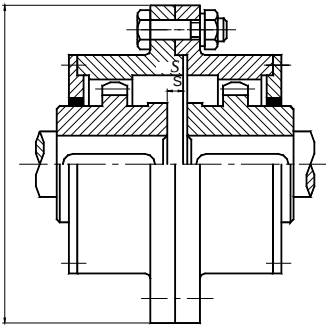
图17 齿式联轴器
