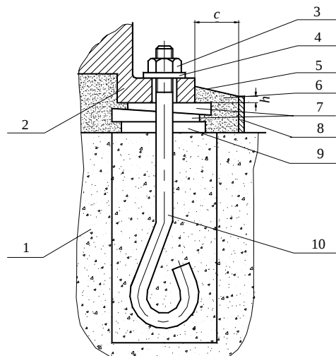
1 - 基础; 2 - 底座底面; 3 - 螺母; 4 - 垫圈; 5 - 灌浆层斜面; 6 - 灌浆层; 7 - 成对斜垫铁; 8 - 外模板; 9 - 平垫铁; 10 - 地脚螺栓
