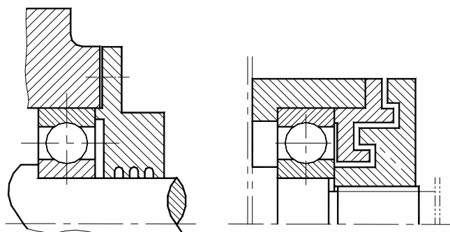
a) 防尘节流环密封
