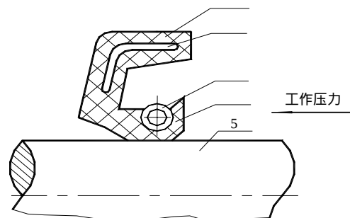
1 - 橡胶皮碗；2 - 金属骨架；3 - 拉紧弹簧；4 - 密封唇部；5 - 主轴
