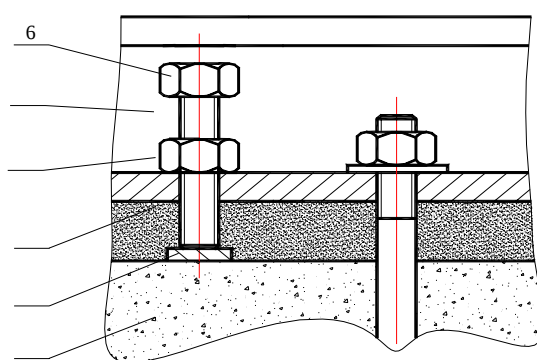
1 - 基础；2 - 垫板；3 - 二次灌浆层；4 - 固定螺母；5 - 机器底座；6 - 顶丝
