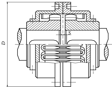
图21 蛇形弹簧联轴器
