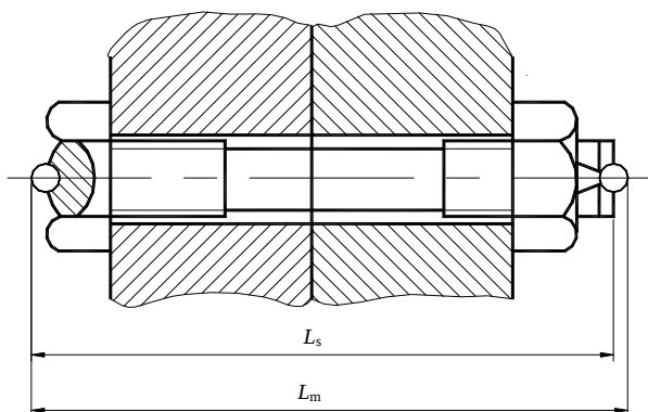
图5 伸长后的螺栓
