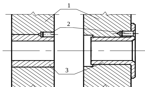
1 - 轴承体; 2 - 固定螺钉; 3 - 轴承
