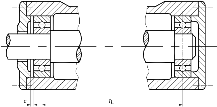
图7 轴承装配间隙
