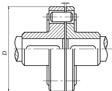
图19 弹性柱销联轴器
