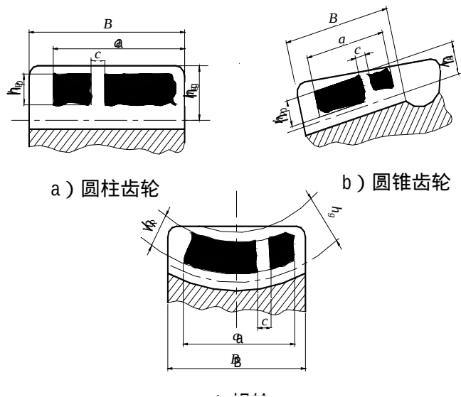
图23 着色法检查传动齿轮、蜗轮啮合的接触斑点
