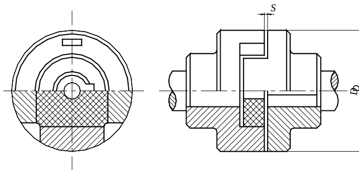
图16 滑块联轴器
