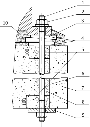
1 - 地脚螺栓；2 - 螺母、垫圈；3 - 底座；4 - 垫铁组；5 - 砂浆层；6 - 预留孔； 7 - 基础；8 - 砂填充层；9 - 锚板；10 - 二次灌浆层
