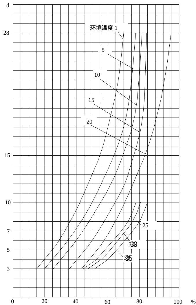
图E.1 混凝土强度增长率
