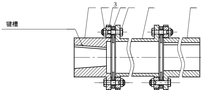
1、7 - 安装盘；2 - 自锁螺母；3 - 衬套；4 - 叠片组件；5 - 螺栓；6 - 间隔轴
