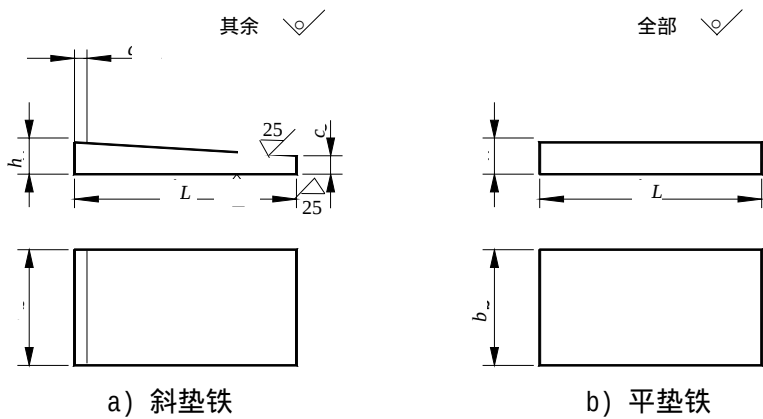
图1 垫铁
