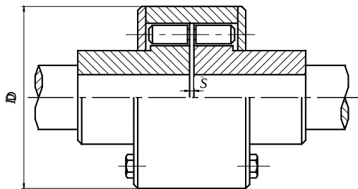
图20 弹性柱销齿式联轴器
