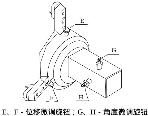
图G.2 激光发射器示意
