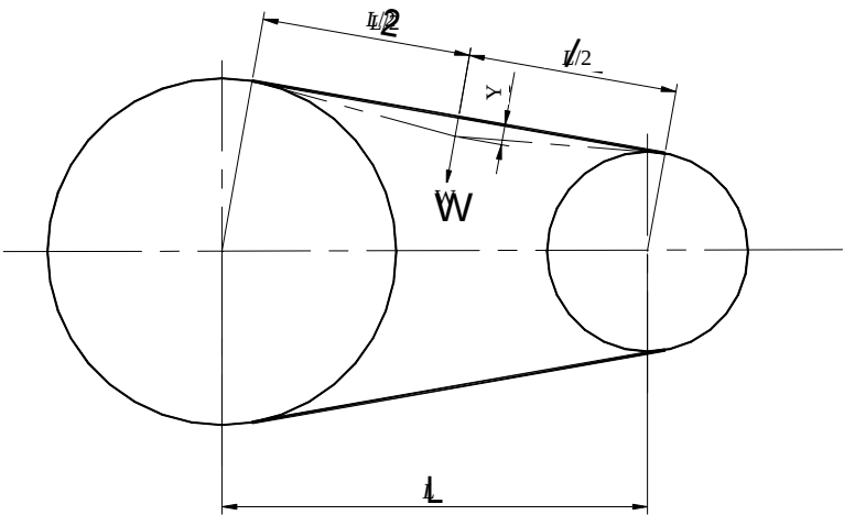
图N.1 皮带拉紧力的测定示意
