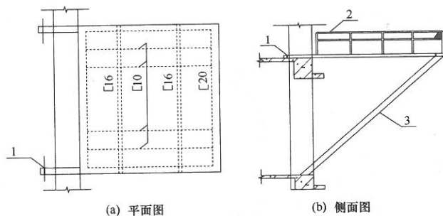
图 C.0.1-2 下支承方式的悬挑式操作平台示意图 (单位: mm) 1—梁面预埋件; 2—栏杆与 [16 焊接; 3—斜撑杆
